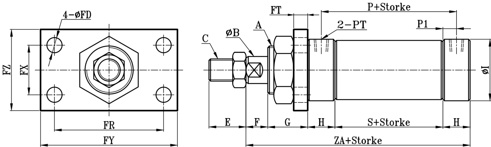
SOA:SOA+FA(圓型-共用) TYPE
